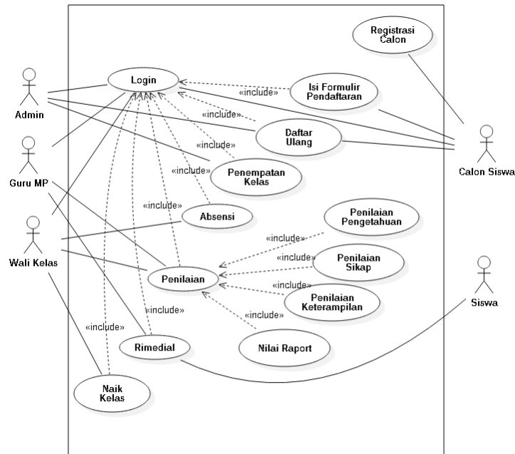
Gambar 1. Use case sistem informasi akademik
