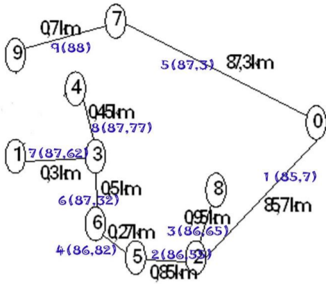
Gambar 7. Pembentukan MST dengan Algoritma Dijkstra pada kasus 2
