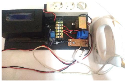
Gambar 4. Perancangan Mekanik Sistem
