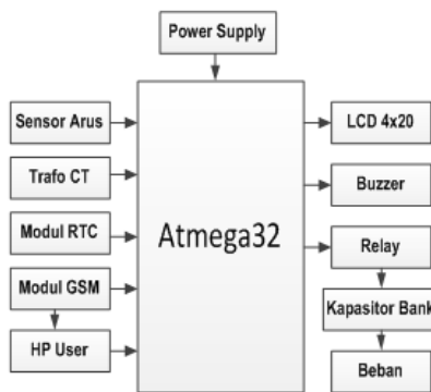
Gambar 5. Diagram Blok Perangkat Keras ( Hardware ) Secara Keseluruhan
