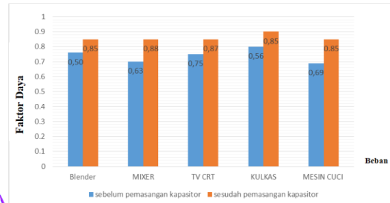
Gambar 12. Grafik Perbandingan Nilai Faktor Daya
