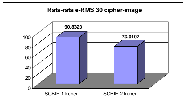
Gambar 2 Grafik perbandingan e_{rms}
